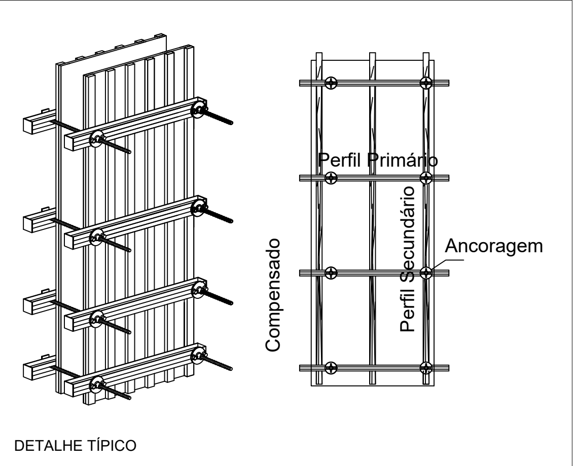
DETALHE TÍPICO
